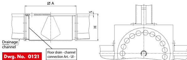
Dwg. No. 0121
