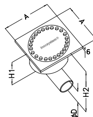
Inoxsystem® IDrain 0010 - Siphon de sol avec plaque carrée pleine de 6 mm avec trous sortie horizontale siphonnée - panier amovible
