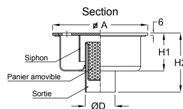
Inoxsystem® IDrain 0013 - Siphon de sol avec plaque carrée pleine de 6 mm avec trous sortie verticale siphonnée - panier amovible
