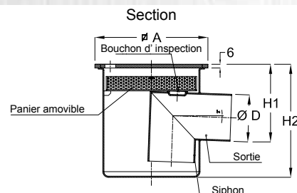
Inoxsystem® IDrain 0011 - Siphon de sol avec plaque carrée pleine de 6 mm avec trous sortie horizontale hyper-surbaissée, siphonnée - panier amovible
