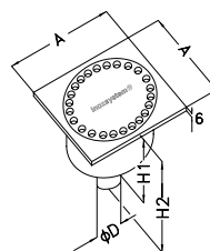
Inoxsystem® IDrain 0013 - Siphon de sol avec plaque carrée pleine de 6 mm avec trous sortie verticale siphonnée - panier amovible
