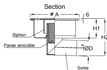
Inoxsystem® IDrain 0010 - Siphon de sol avec plaque carrée pleine de 6 mm avec trous sortie horizontale siphonnée - panier amovible
