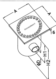
Inoxsystem® IDrain 0011 - Siphon de sol avec plaque carrée pleine de 6 mm avec trous sortie horizontale hyper-surbaissée, siphonnée - panier amovible
