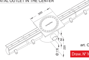
art. CFOT ..... Draw. N° 1052 - 14
