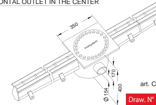
art. CFOTCG ..... Draw. N° 2252 - 14
