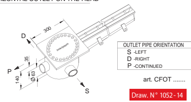
art. CFOT ..... Draw. N° 1052 - 14
