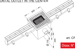
art. CFOTS ..... Draw. N° 1062 - 14
